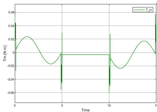
Figura 102: Torque T_m con controlador discreto codificado
